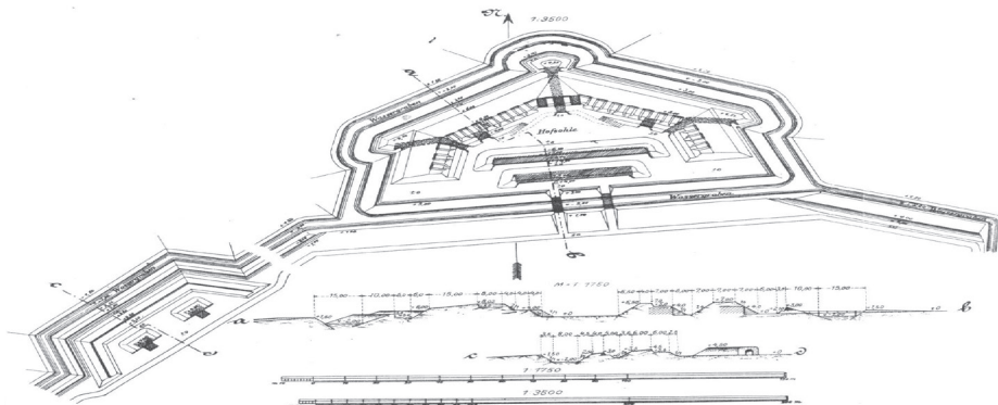
Skizze eines ehem. russ. Forts (Fort II von Ossowec)
